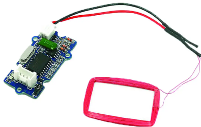
Lecteur RFID branché sur D6
